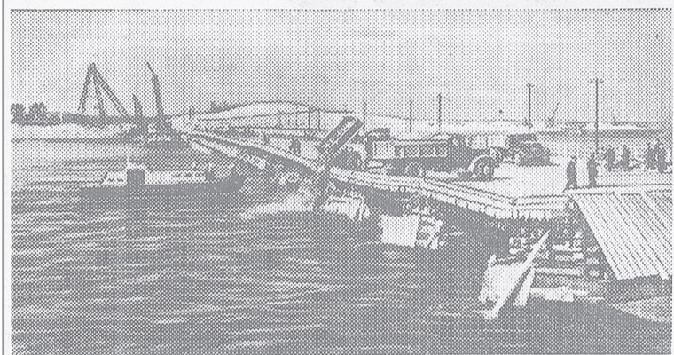
Для перекрытия русла Волги на строительстве Горьковской гидроэлектростанции сооружен понтонный мост шириной в 20 метров и длиной в 300 метров, с которого автосамосвалы сбрасывают камень. На снимке общий вид понтонного моста.
